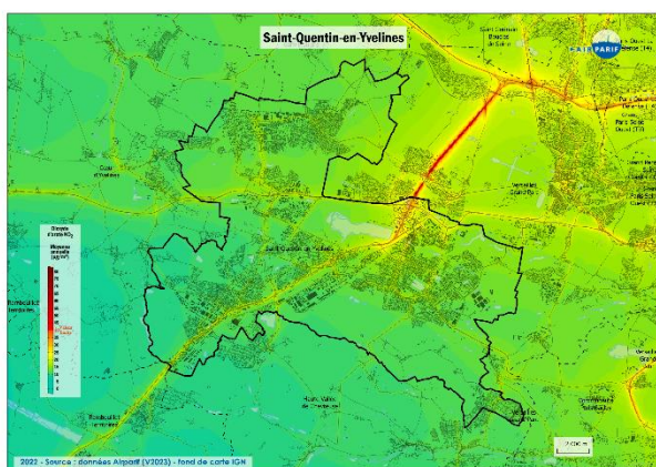
Concentration moyenne annuelle en NO 2 dans le territoire de Saint-Quentin-en-Yvelines et dans les Yvelines en 2022.
