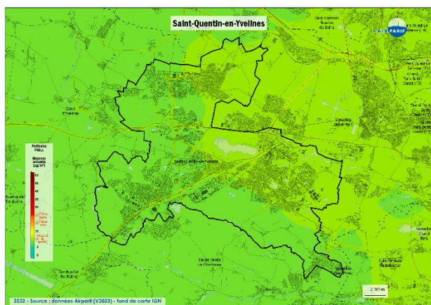
Concentration moyenne annuelle en PM 2.5 dans le territoire de Saint-Quentin-en-Yvelines et dans les Yvelines en 2022
