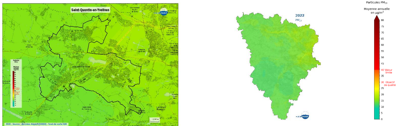
Concentration moyenne annuelle en PM 10 dans le territoire de Saint-Quentin-en-Yvelines et dans les Yvelines en 2022
