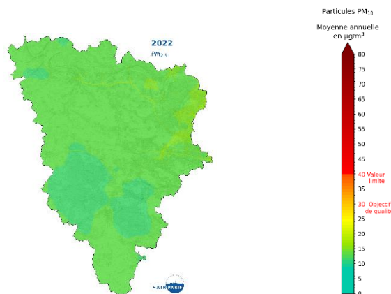
Concentration moyenne annuelle en PM 2.5 dans le territoire de Saint-Quentin-en-Yvelines et dans les Yvelines en 2022
