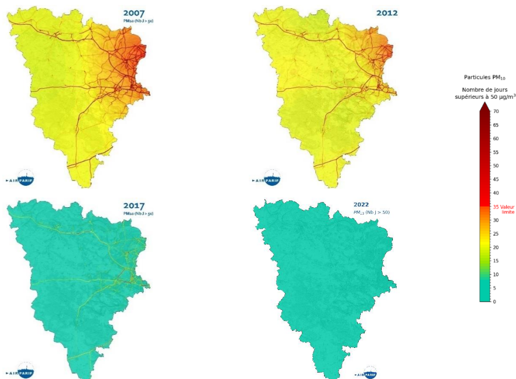
Nombre de jours de dépassement du seuil journalier de 50 \mu\text{g}/\text{m}^3 en \text{PM}_{10} de 2007 à 2022 dans les Yvelines
