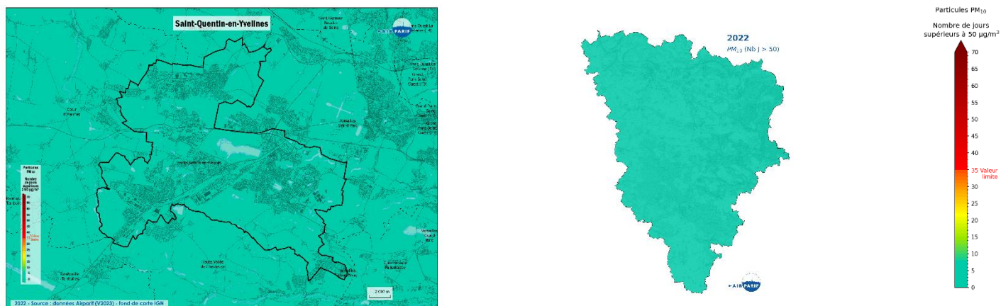
Nombre de jours de dépassement du 50 µg/m 3 en PM 10 dans le territoire de Saint-Quentin-en-Yvelines et dans les Yvelines en 2022.
