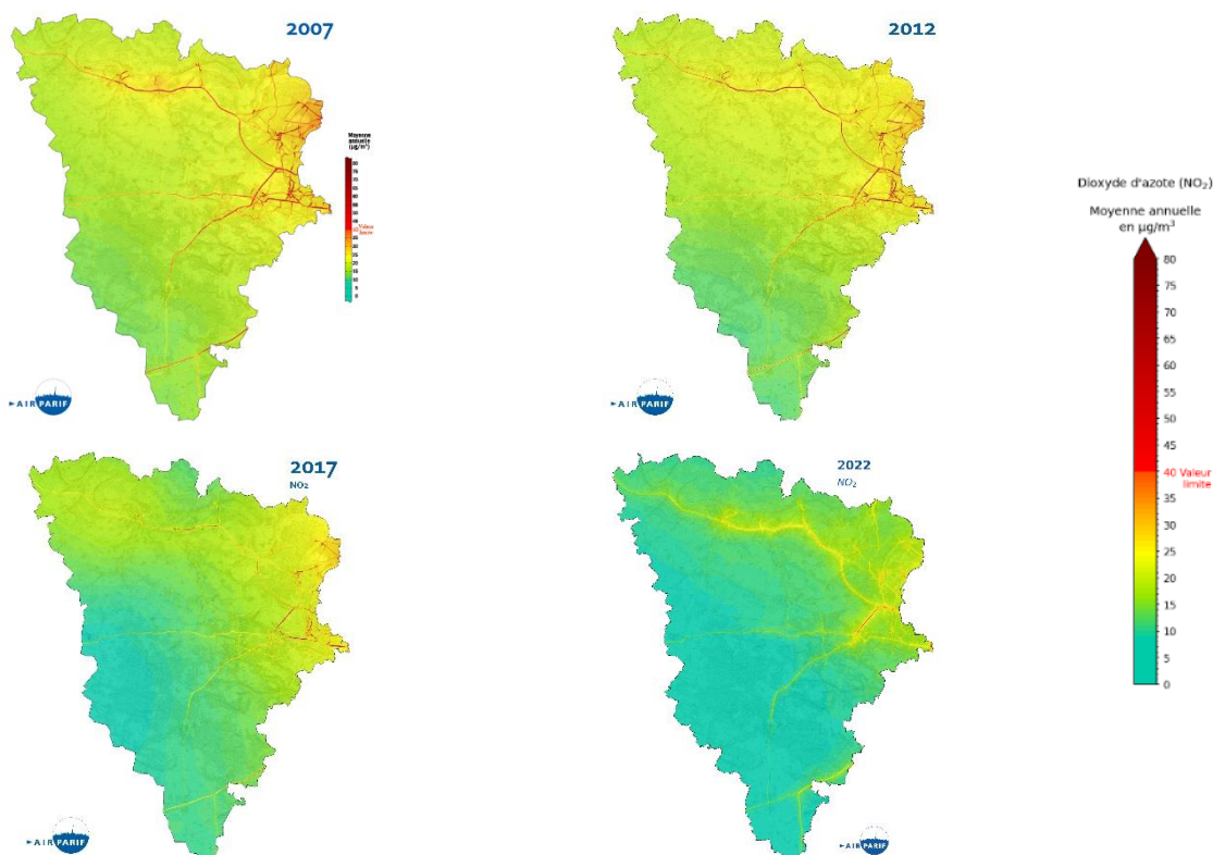
Évolution de la moyenne annuelle en NO 2 de 2007 à 2022 dans les Yvelines.
