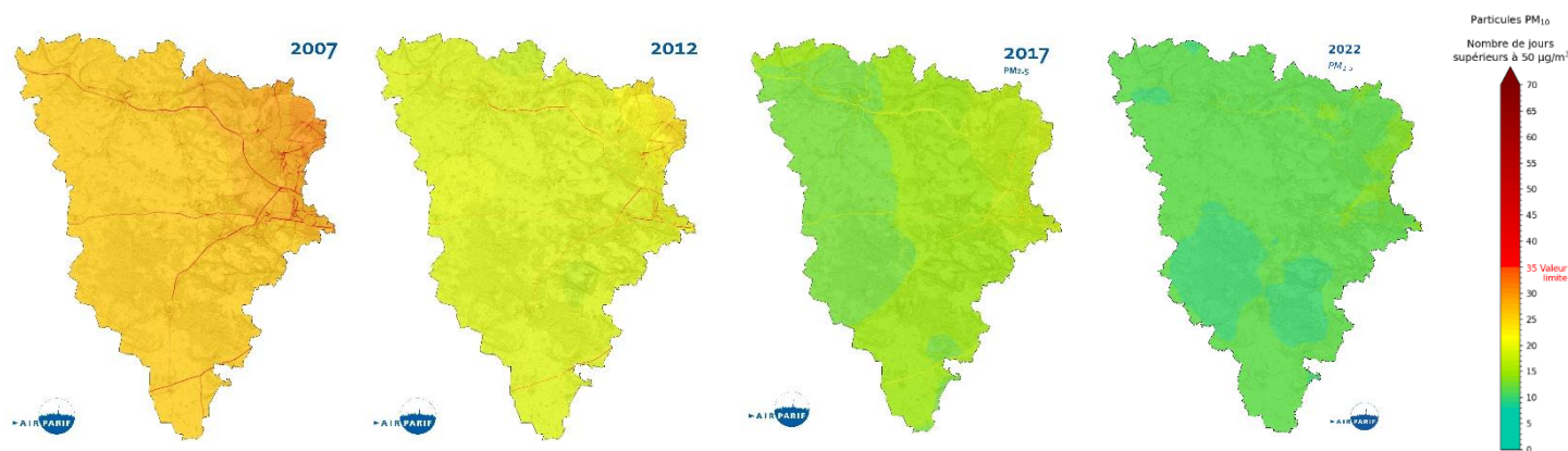
Evolution de la moyenne annuelle en PM 2.5 de 2007 à 2022 dans les Yvelines
