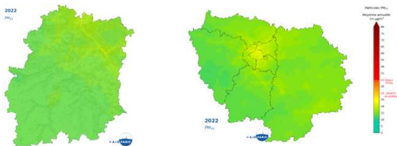
Concentration moyenne annuelle en PM 10 dans l'Essonne et en Ile-de-France en 2022
