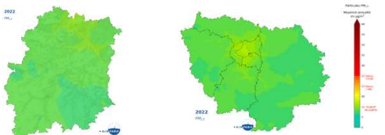
Concentration moyenne annuelle en PM 2.5 dans l'Essonne et en Ile-de-France en 2022
