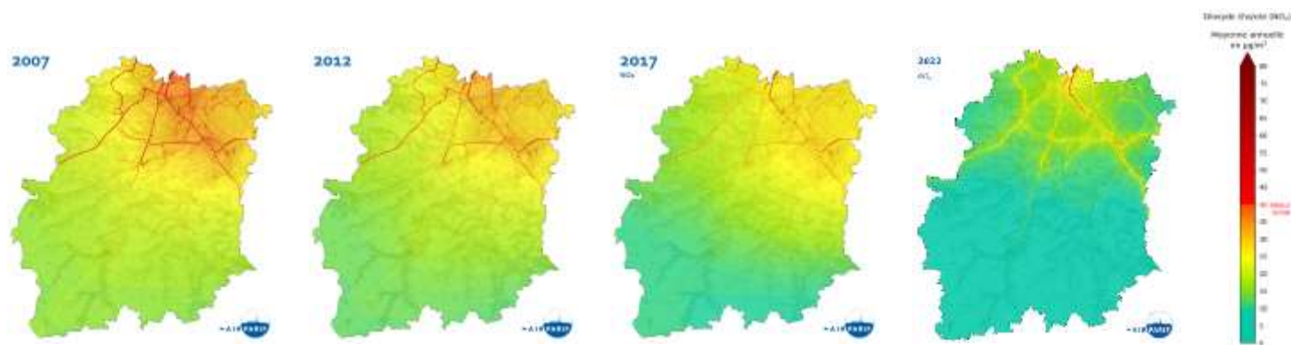
Évolution de la moyenne annuelle en NO 2 de 2007 à 2022 dans l'Essonne
