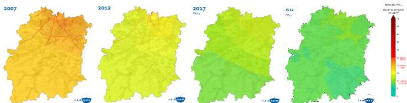
Évolution de la moyenne annuelle en PM 2.5 de 2007 à 2022 dans l'Essonne
