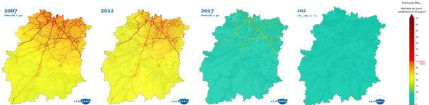
Nombre de jours de dépassement du seuil journalier de 50 \mu\text{g}/\text{m}^3 en \text{PM}_{10} de 2007 à 2022 dans l'Essonne
