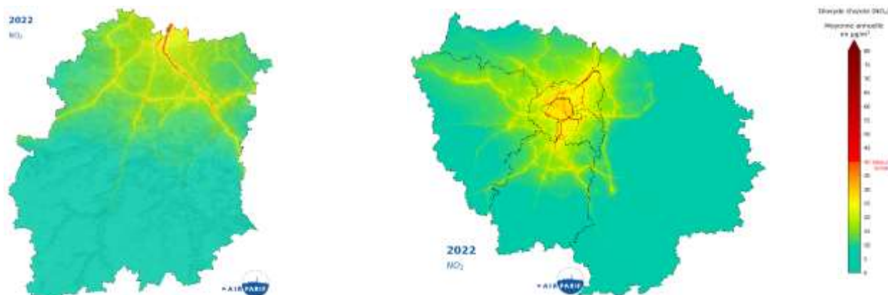
Concentration moyenne annuelle en NO 2 dans l'Essonne et en Ile-de-France en 2022.
