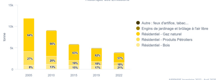
NOx - Ile-de-France Historique des Emissions
