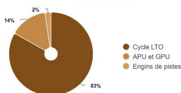
Répartition des émissions des Plateformes aéroportuaires - GES
