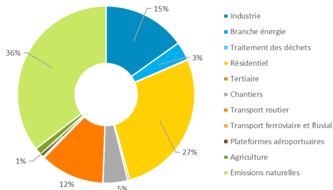
COVNM - IDF - 2022 - Hiver
