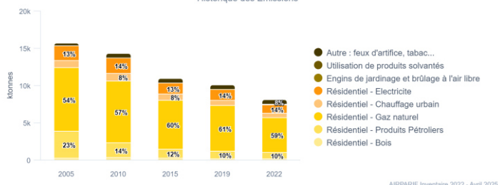
GES scope 1+2 - Ile-de-France Historique des Emissions
