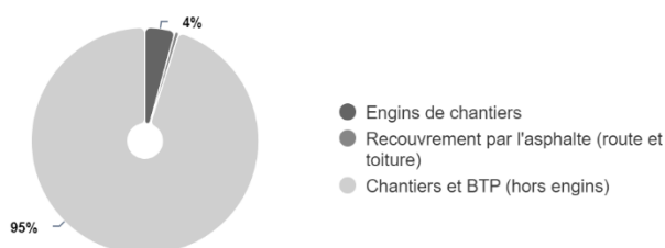
Répartition des émissions des chantiers - PM 10
