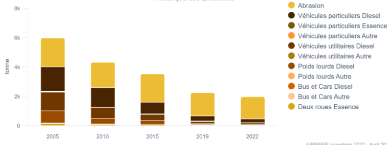
PM 2.5 - Ile-de-France Historique des Emissions
