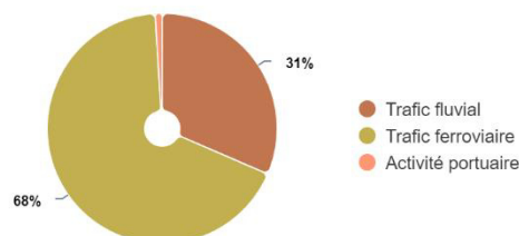
Répartition des émissions des autres transports - PM 2.5
