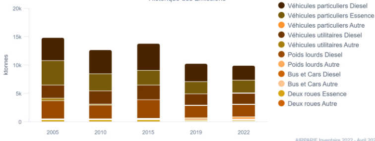
GES scope 1+2 - Ile-de-France Historique des Emissions
