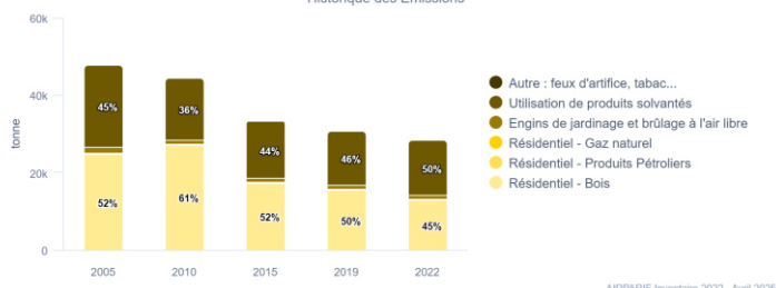
COVNM - Ile-de-France Historique des Emissions
