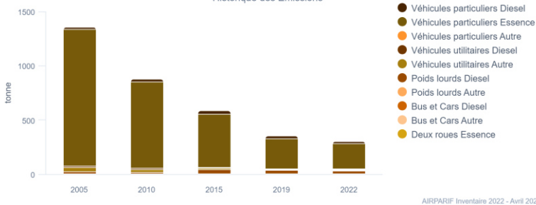
NH 3 - Ile-de-France Historique des Emissions
