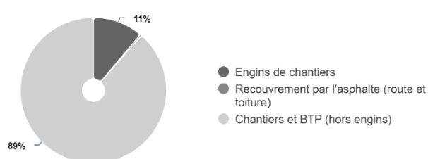
Répartition des émissions des chantiers - PM 2.5
