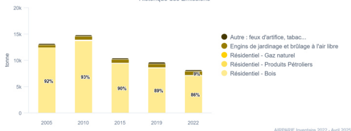
PM 10 - Ile-de-France Historique des Emissions
