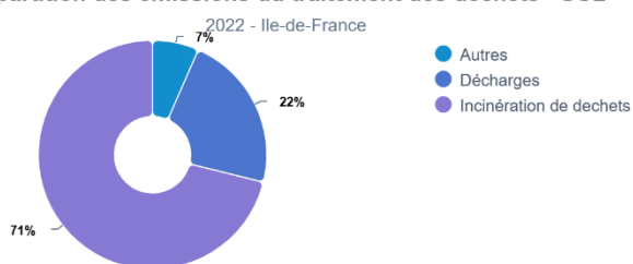
Répartition des émissions du traitement des déchets - SO 2
