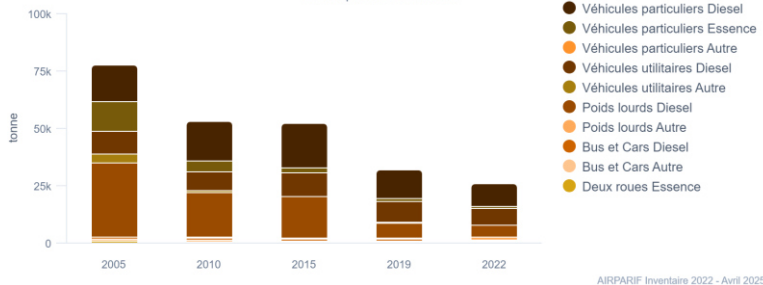
NO x - Ile-de-France Historique des Emissions
