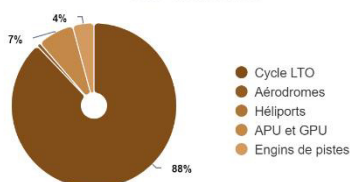
Répartition des émissions des Plateformes aéroportuaires - NOx
